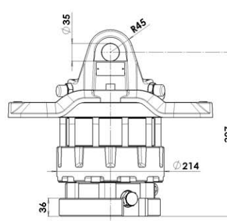
FR 110F DH
