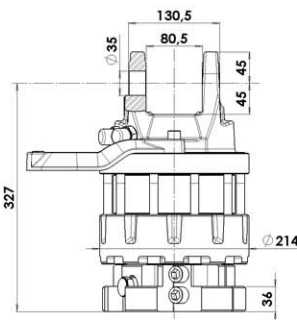
FR 110F SH
